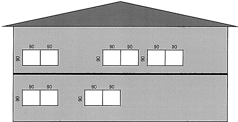
南立面图
