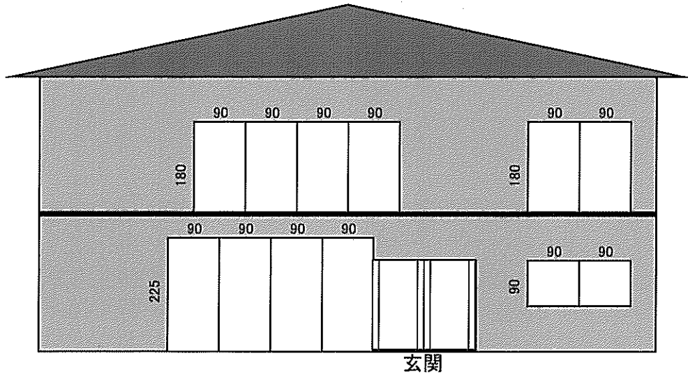
北立面图
