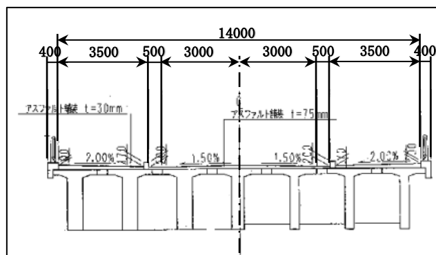
橋梁断面図
