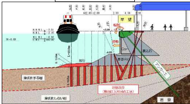
岸壁の整備断面図
