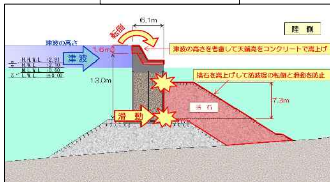
防波堤の整備断面図
