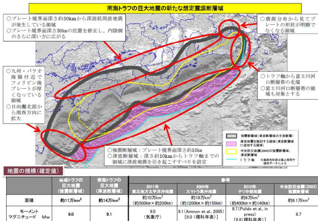
南海トラフ巨大地震の想定震源断層域
