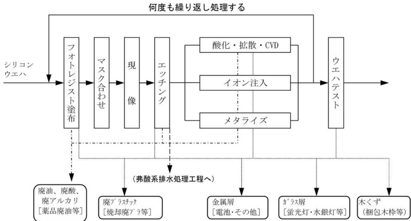
図 1. ウェハ製造工程フローシート [NO. 1]
